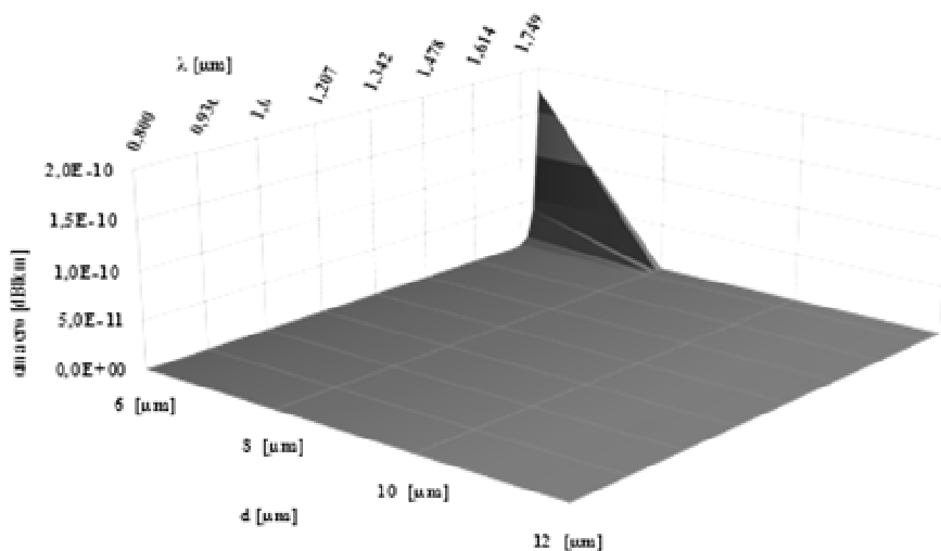
Фигура 5 Загуби от Макроогъвания на влакно със стъпално-радиален профил d=6\mu\text{m} \div 12\mu\text{m} , \Delta=0.01
