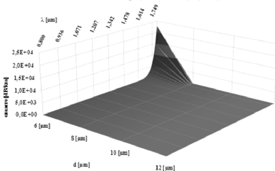
Загуби от Макроогъвания на влакно с градиентно-радиален профил: g=2 , d=6\mu\text{m} \div 12\mu\text{m} , \Delta=0.01
