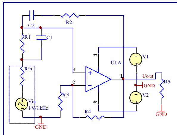
Фиг.1. Принципна схема на филтър с мост на Вин
