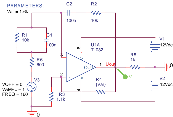
Фиг. 2. Принципно схема за провеждане на числен експеримент с програмнен продукт OrCAD
