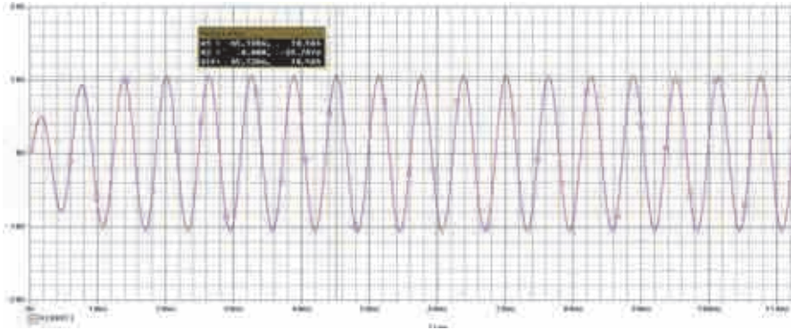
Фиг. 4. Ограничение на максималната изходна амплитуда при стойност на R4=1.6k\Omega
