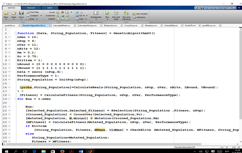
Фигура 3. Част от изходния сорс-код на GeneticAlgorithm20
