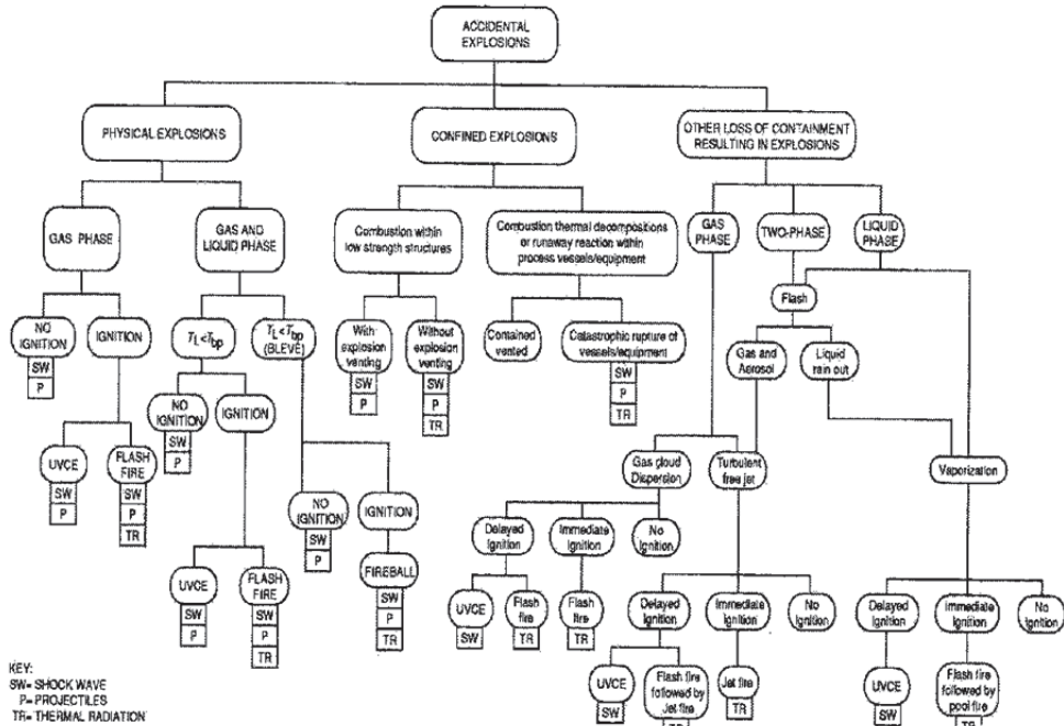
Фиг. 4. Дърво на събитията
