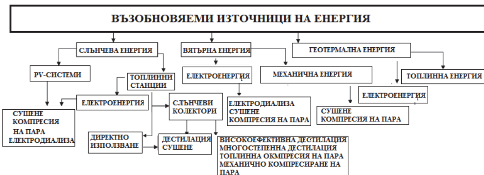
Фиг. 2. Възможни технологични комбинации на основните възобновяеми източници на енергия и методите за опресняване на вода.
