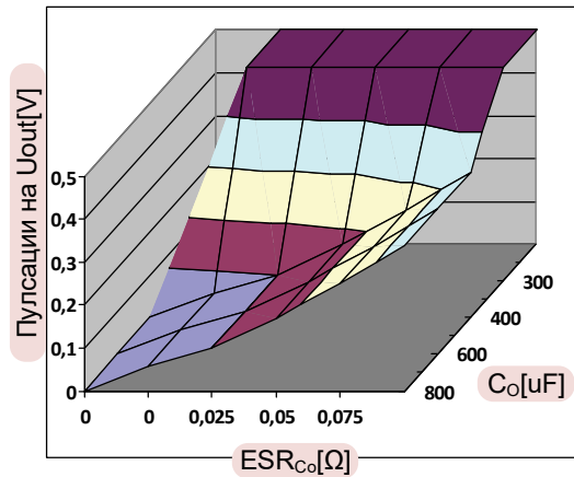
Фиг. 3. Зависимост на пулсациите на изходното напрежение от еквивалентното последователно съпротивление ( ESR_{Co} ) на изходния кондензатор
