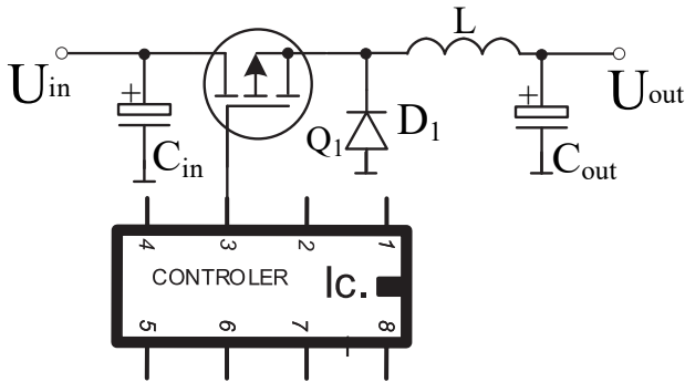
Фиг. 1. Основна схема на понижаващ преобразувател
